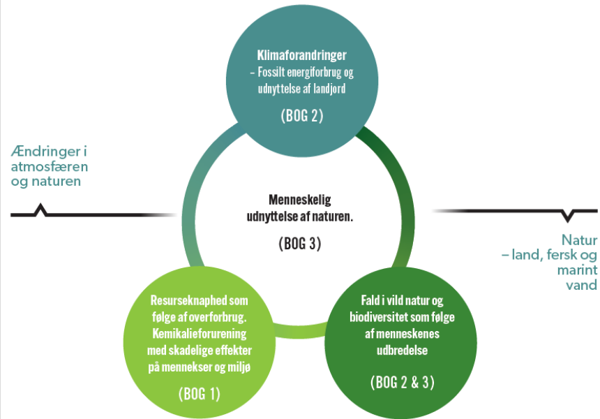
Figur 1 Anthropocæne Tidsalder.
